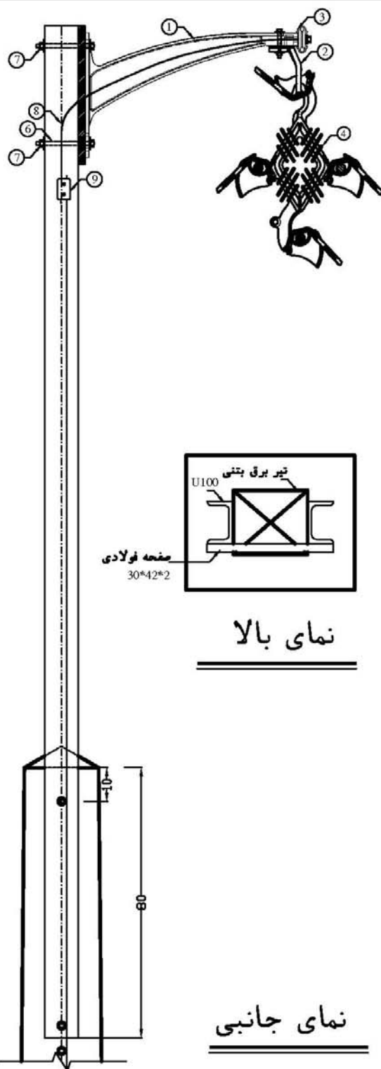
نمای روبرو
