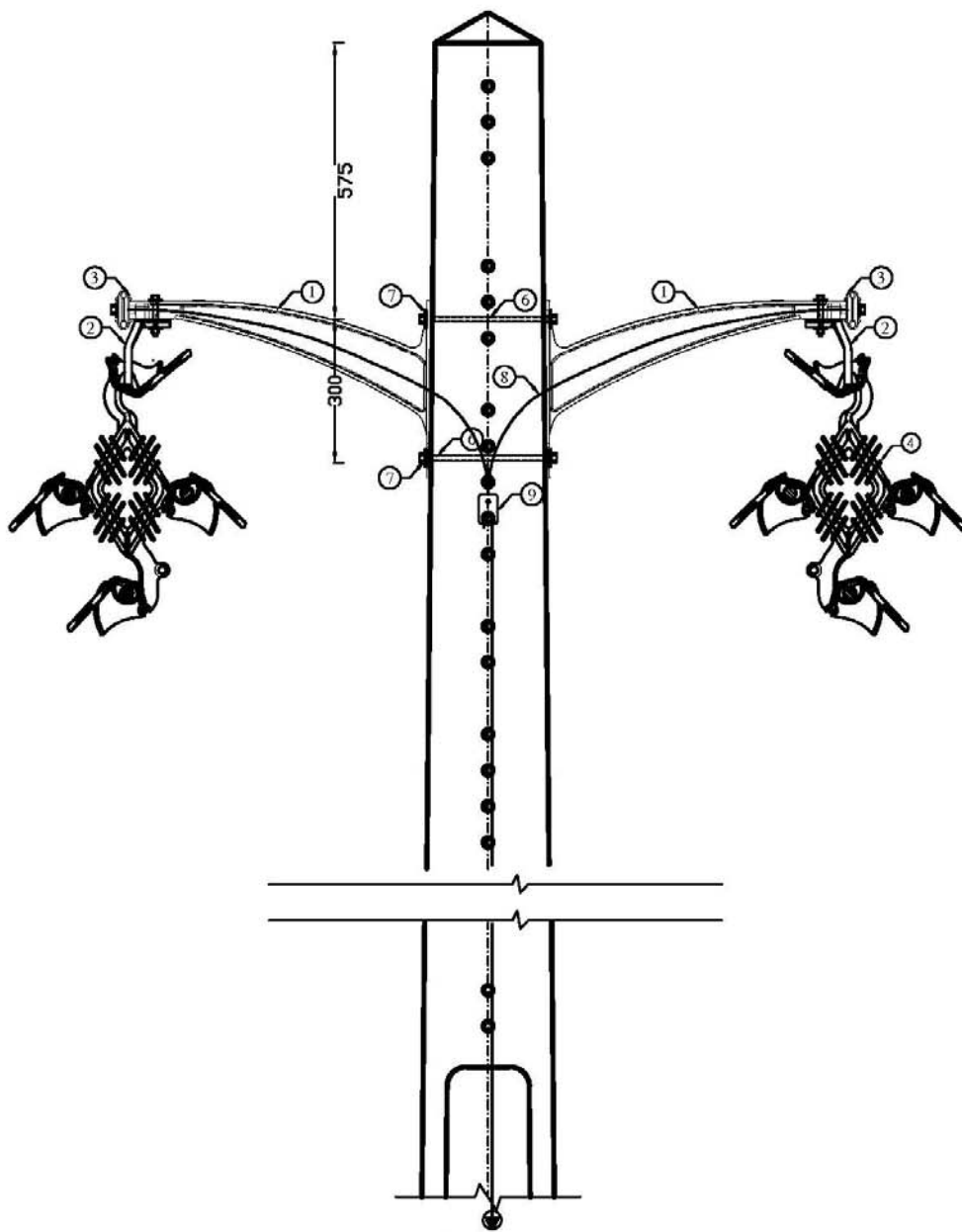
نمای جانبی
